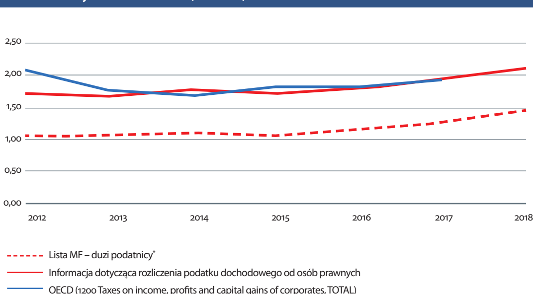
Podatek należny CIT do PKB w Polsce (dane w %)
