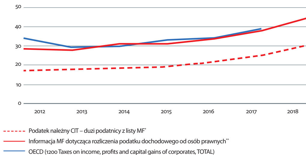
Podatek należny CIT (dane w mld zł)
