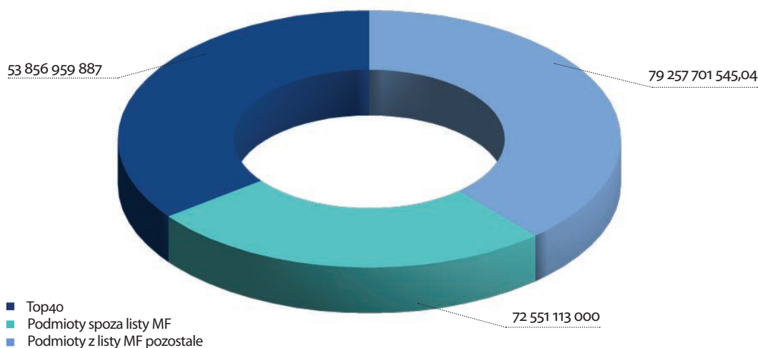
Udział w dochodach w CIT w latach 2013–2018
